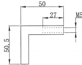
DS Fixing Bolt 2PCS
